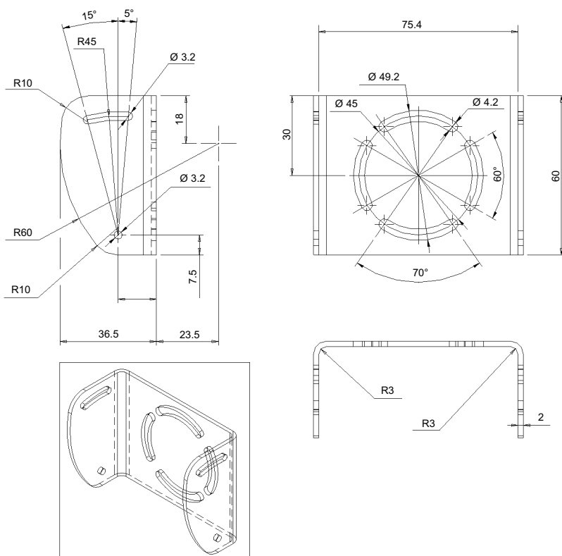
ST-5048 Equerre de fixation angulaire ajustable
