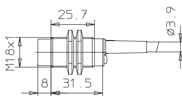
E2EL-X8M□ 2M
