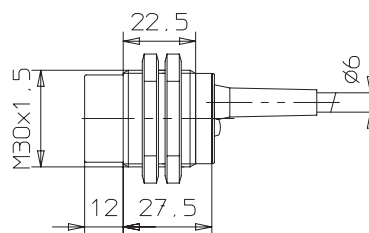
E2EL-X15M□ 2M
