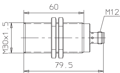
E2EL-X10□-M1L
