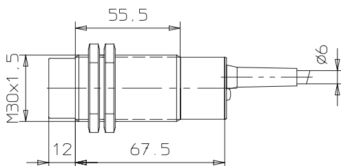
E2EL-X10□-L 2M
