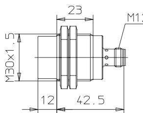
E2EL-X15M□-M1
