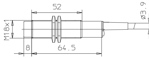
E2EL-X8M□-L 2M
