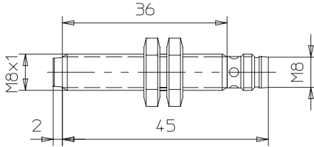
E2EL-X2M□-M3
