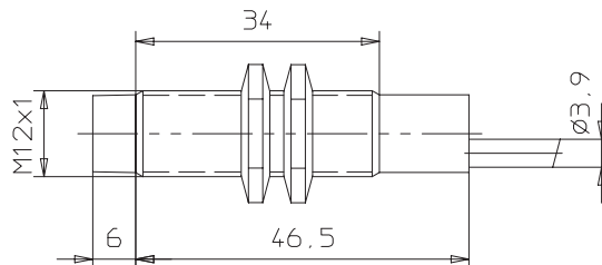
E2EL-X4M□-L 2M
